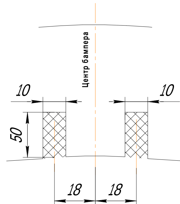
Вид С
